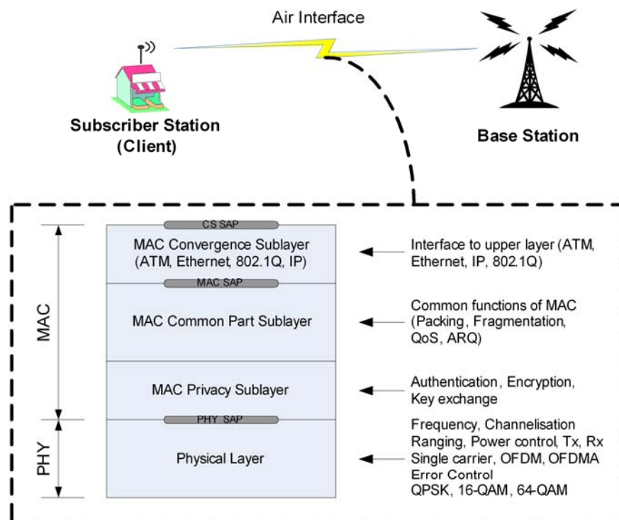
รูปที่ 3 IEEE 802.16 Protocol Stack
