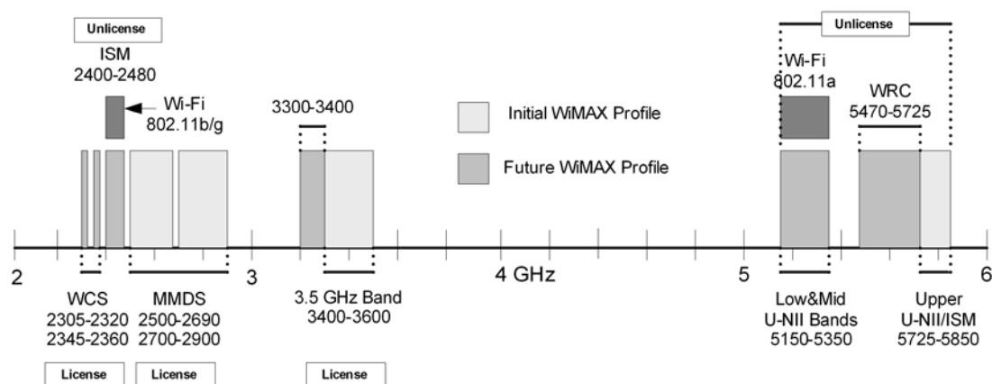
รูปที่ 14 WiMAX Spectrum
