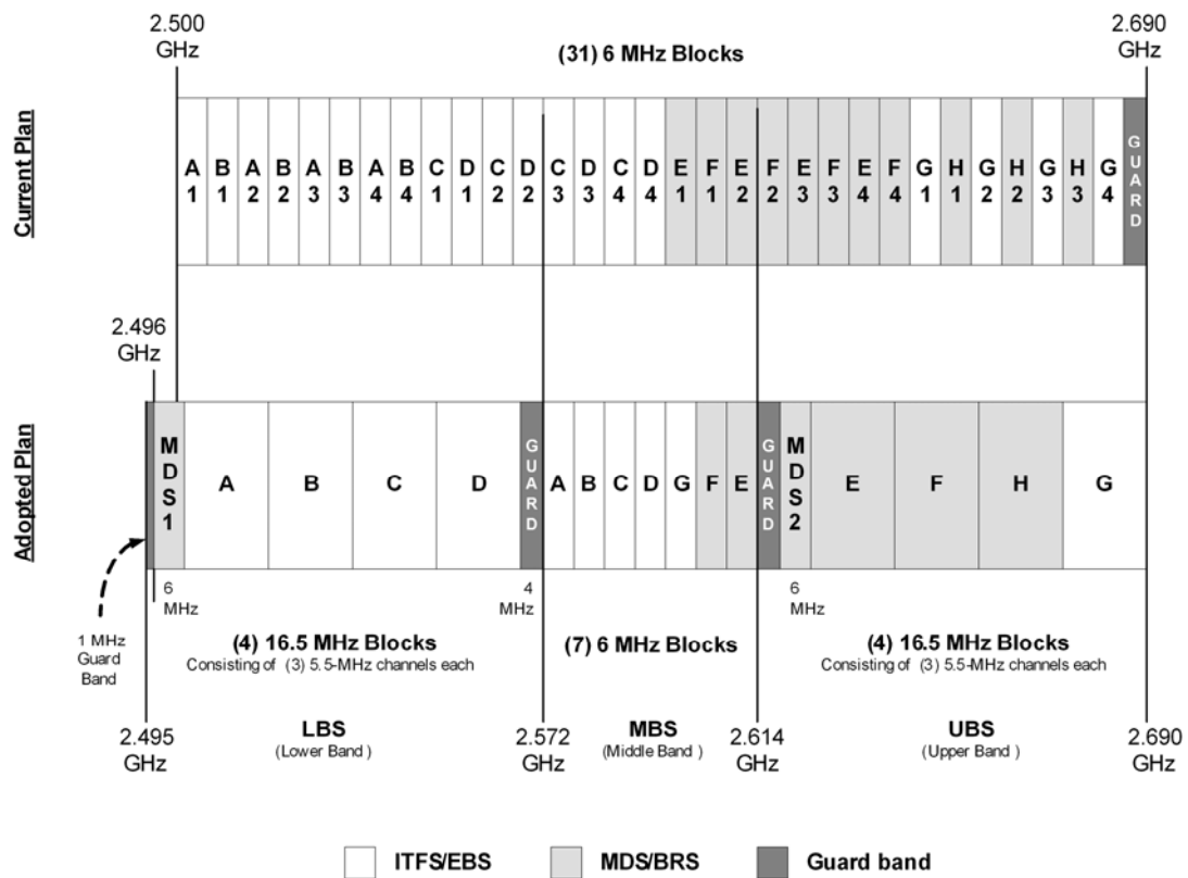
รูปที่ 20 การจัดสรรความถี่ในแถบคลื่นวิทยุ 2.495-2.690 GHz ของประเทศสหรัฐอเมริกา ทั้งแผนปัจจุบันและแผนที่จะมีการเปลี่ยนแปลงใหม่
