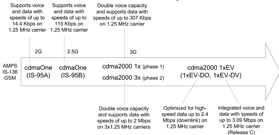
รูปที่ 2 วิวัฒนาการของ cdma2000
