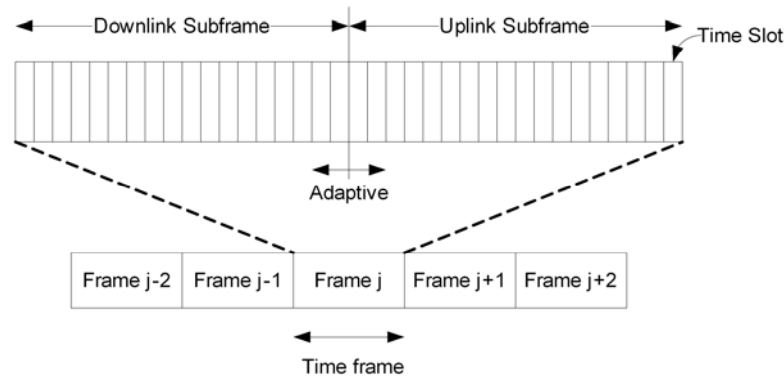
รูปที่ 9 Time Division Duplex (TDD)
