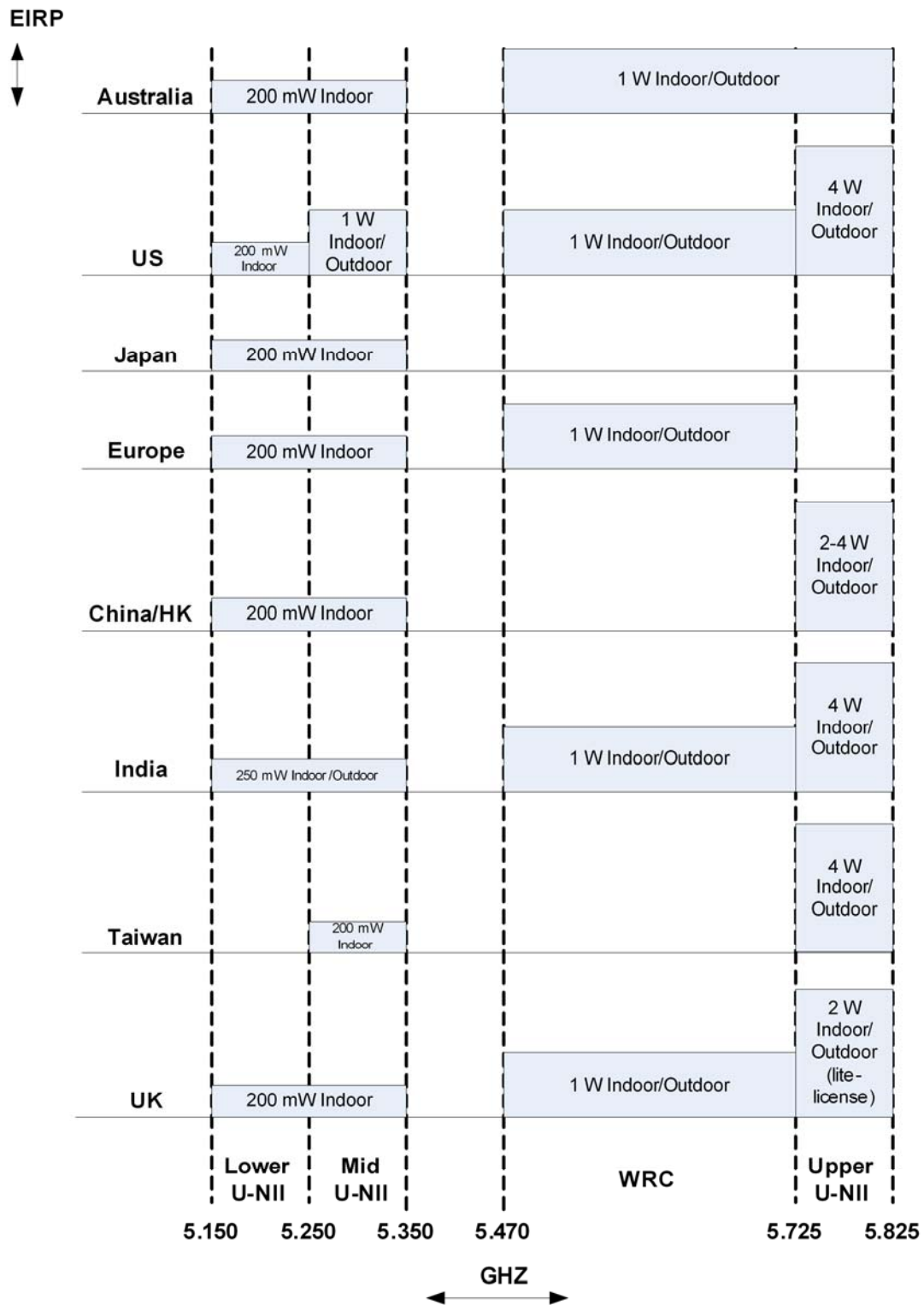
รูปที่ 15 5 GHz Unlicensed Spectrum Allocation ของประเทศต่างๆ
