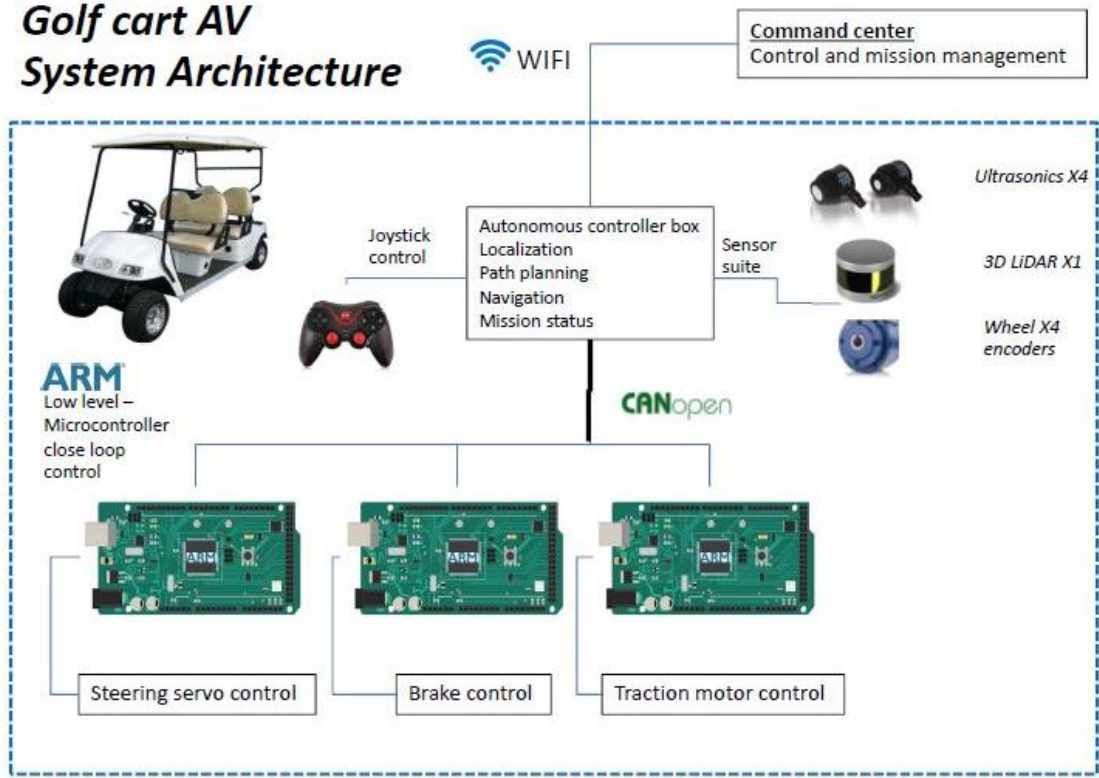
Golfcart AV Prototype – System Architecture
