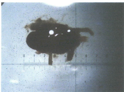
Opiliones: harvestman
