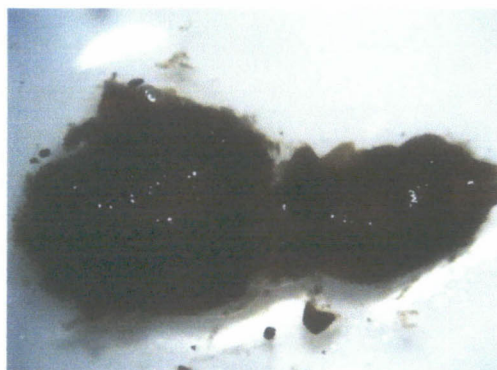
Araneae: spiders
