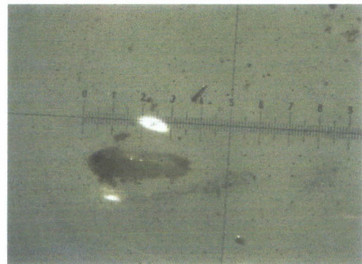
Hemiptera-Homoptera: hopper
