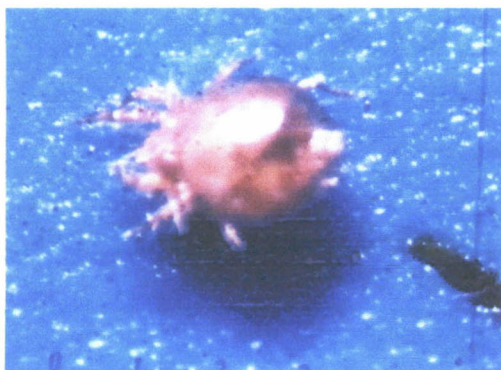
Acari: ticks
